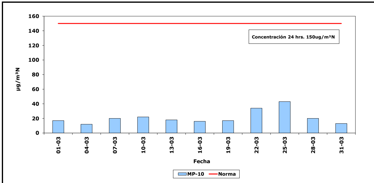
Gráfico N° 1 Concentración de Material Particulado Respirable MP-10 Estación Puerto Mejillones, Marzo 2019
