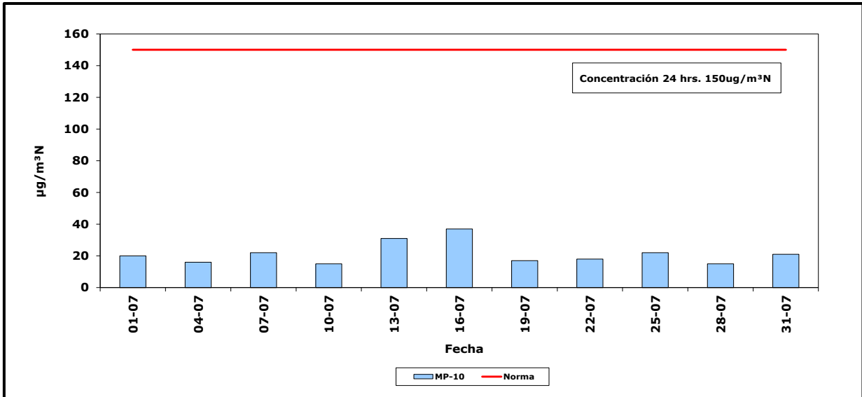
Gráfico N° 1 Concentración de Material Particulado Respirable MP-10 Estación Puerto Mejillones, Julio 2018
