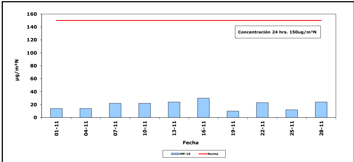
Gráfico N° 1 Concentración de Material Particulado Respirable MP-10 Estación Puerto Mejillones, Noviembre 2018
