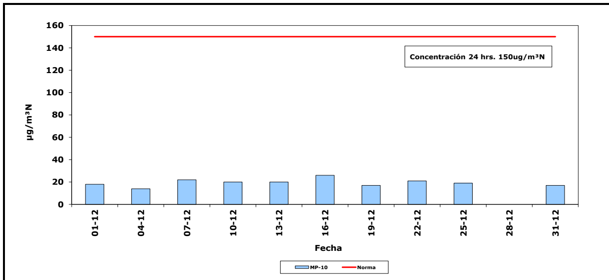
Gráfico N° 1 c Concentración de Material Particulado Respirable MP-10 Estación Puerto Mejillones, Diciembre 2018
