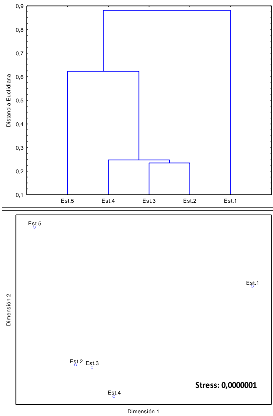
FIGURA 9. PUERTO MEJILLONES. Análisis multidimensional de las variables químicas del estrato PROFUNDO de la columna de agua en las estaciones de muestreo del PSM. MONITOREO JULIO 2016.
