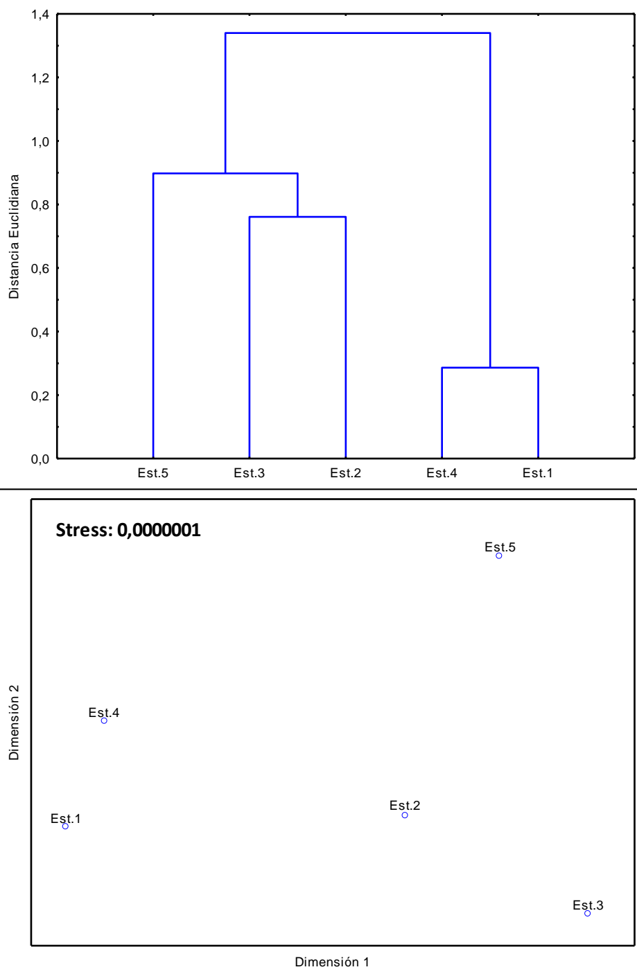
FIGURA 8. PUERTO MEJILLONES. Análisis multidimensional de las variables químicas en el estrato SUPERFICIAL de la columna de agua en las estaciones de muestreo del PSM. MONITOREO JULIO 2016.
