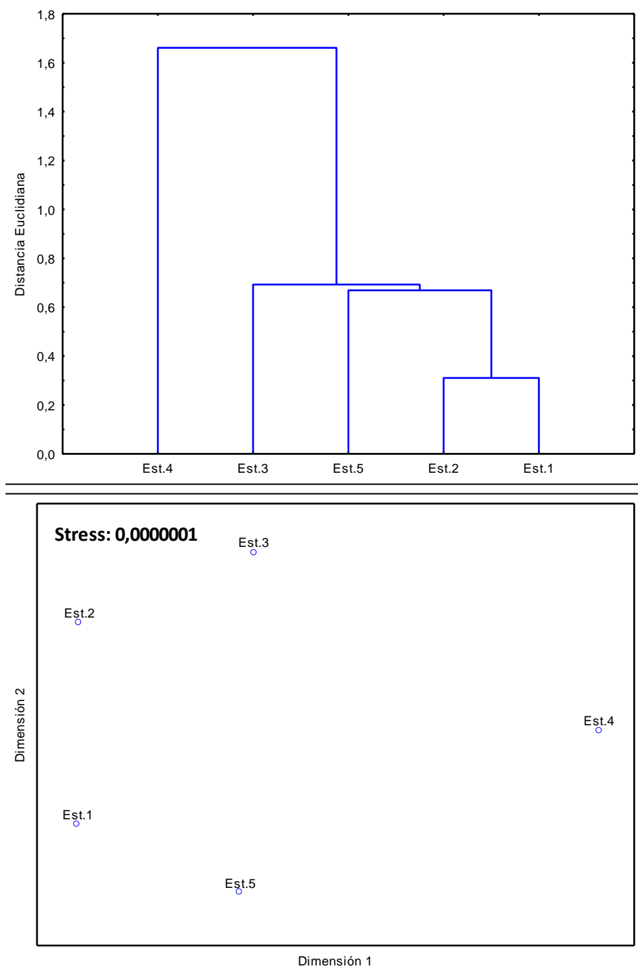
FIGURA 13. PUERTO MEJILLONES. Análisis multidimensional de las variables químicas en biota intermareal ( Emerita analoga ) en las transectas intermareales de muestreo del PSM. MONITOREO JULIO 2016.
