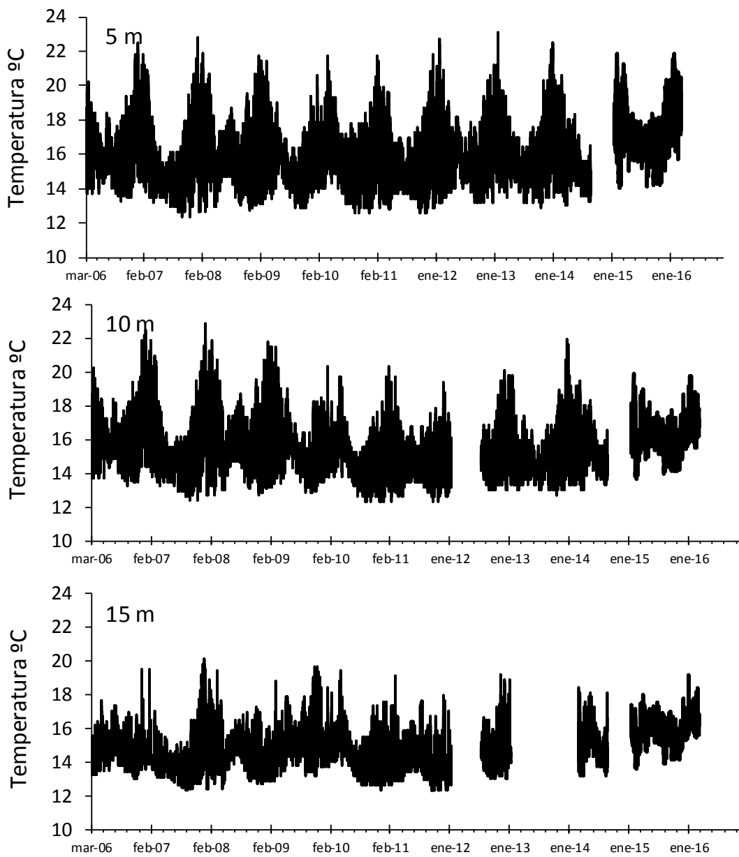
FIGURA 2. PUERTO MEJILLONES. Variación temporal de la temperatura (° C) por estrato de profundidad (m) en el área de estudio del PSM. MONITOREO JULIO 2016.
