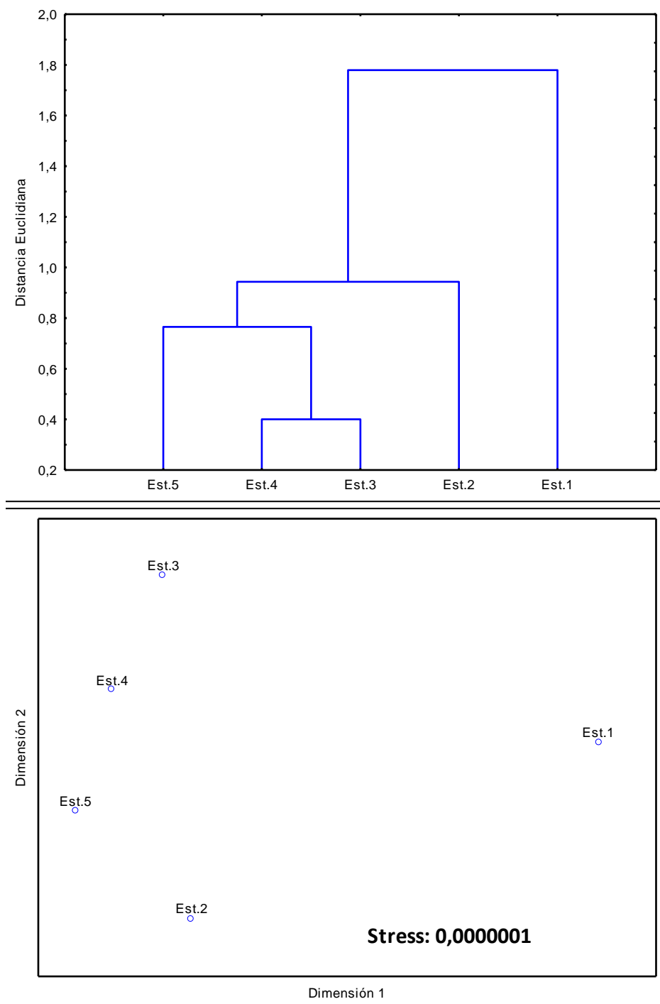
FIGURA 12. PUERTO MEJILLONES. Análisis multidimensional de las variables químicas en los sedimentos de las estaciones submareales en el muestreo del PSM. MONITOREO JULIO 2016.
