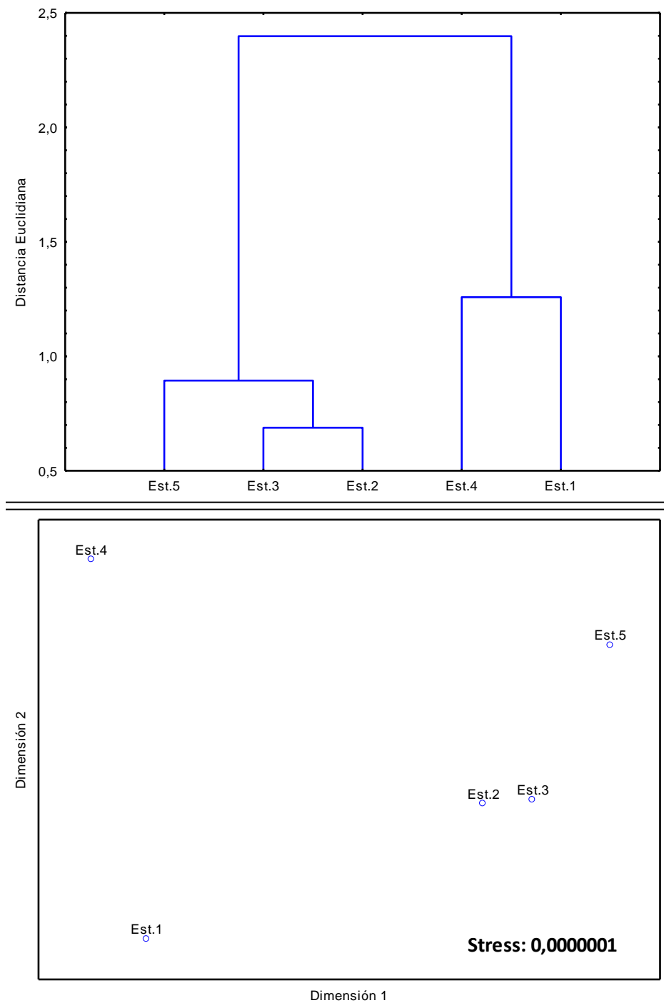
FIGURA 14. PUERTO MEJILLONES. Análisis multidimensional de las variables químicas en biota submareal (moluscos bivalvos) en las estaciones submareales de muestreo del PSM. MONITOREO JULIO 2016.
