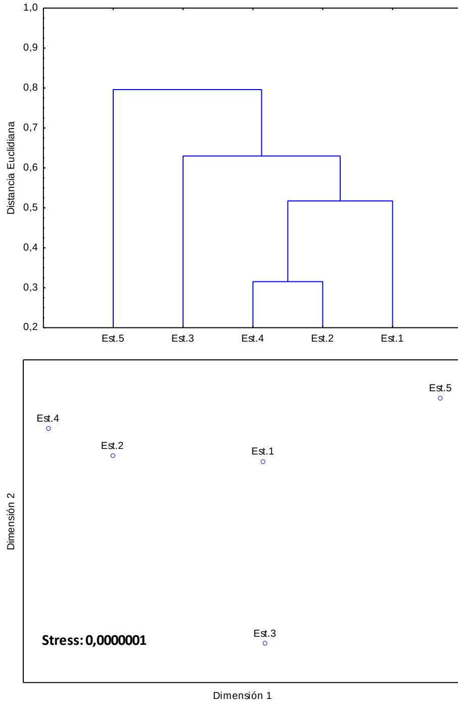
FIGURA 13. PUERTO MEJILLONES. Análisis multidimensional de las variables químicas en biota intermareal ( Emerita analoga ) en las transectas intermareales de muestreo del PSM. MONITOREO MARZO 2014.
