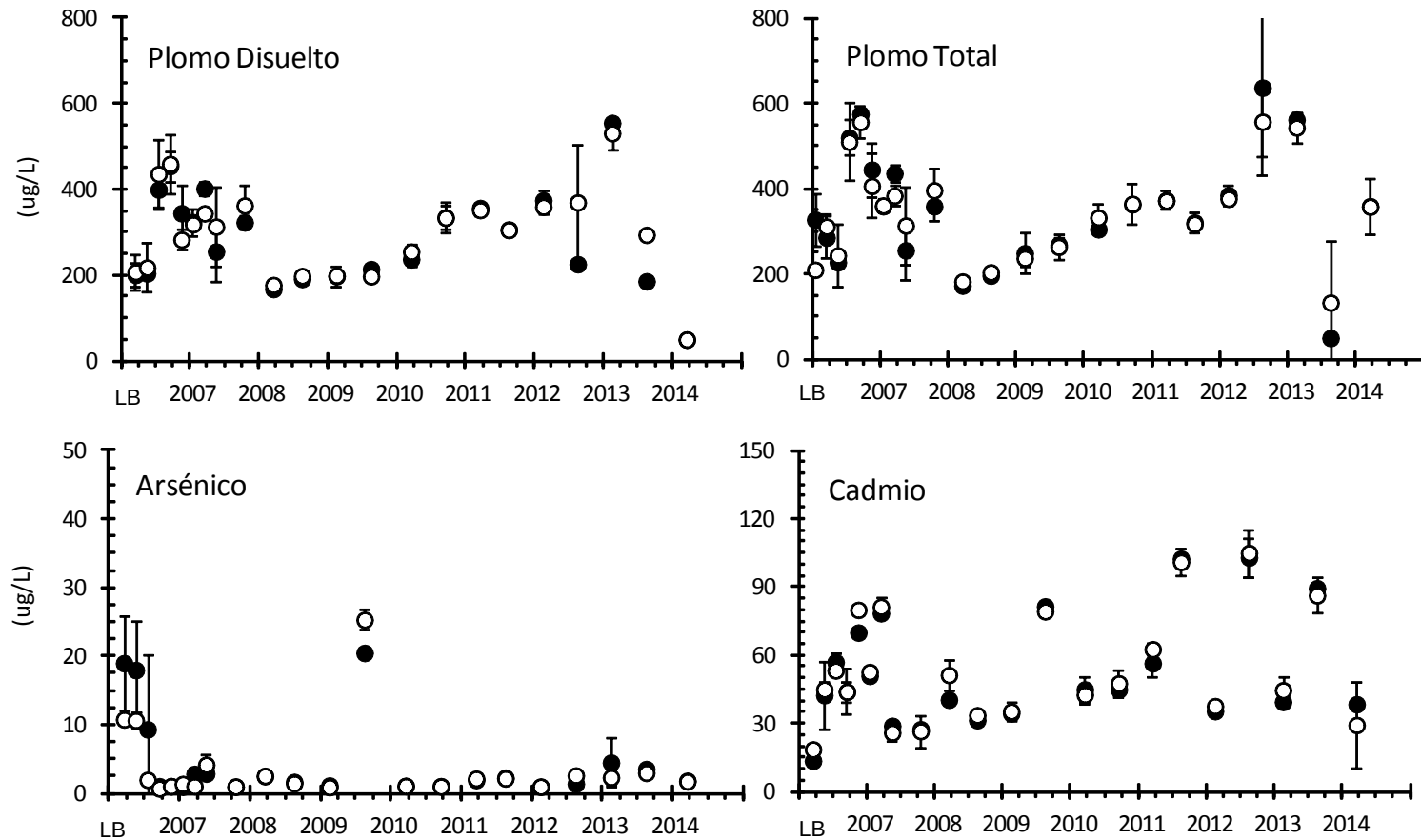
FIGURA 4. PUERTO MEJILLONES. Variabilidad temporal de los parámetros ambientales evaluados en el estrato superficial de la columna de agua de mar. Contraste de la concentración de metales pesados entre estaciones "referenciales y control" (círculos abiertos) y estaciones de monitoreo (círculos cerrados) del PSM. MONITOREO MARZO 2014. Media +/- DS. LB: Línea Base.
