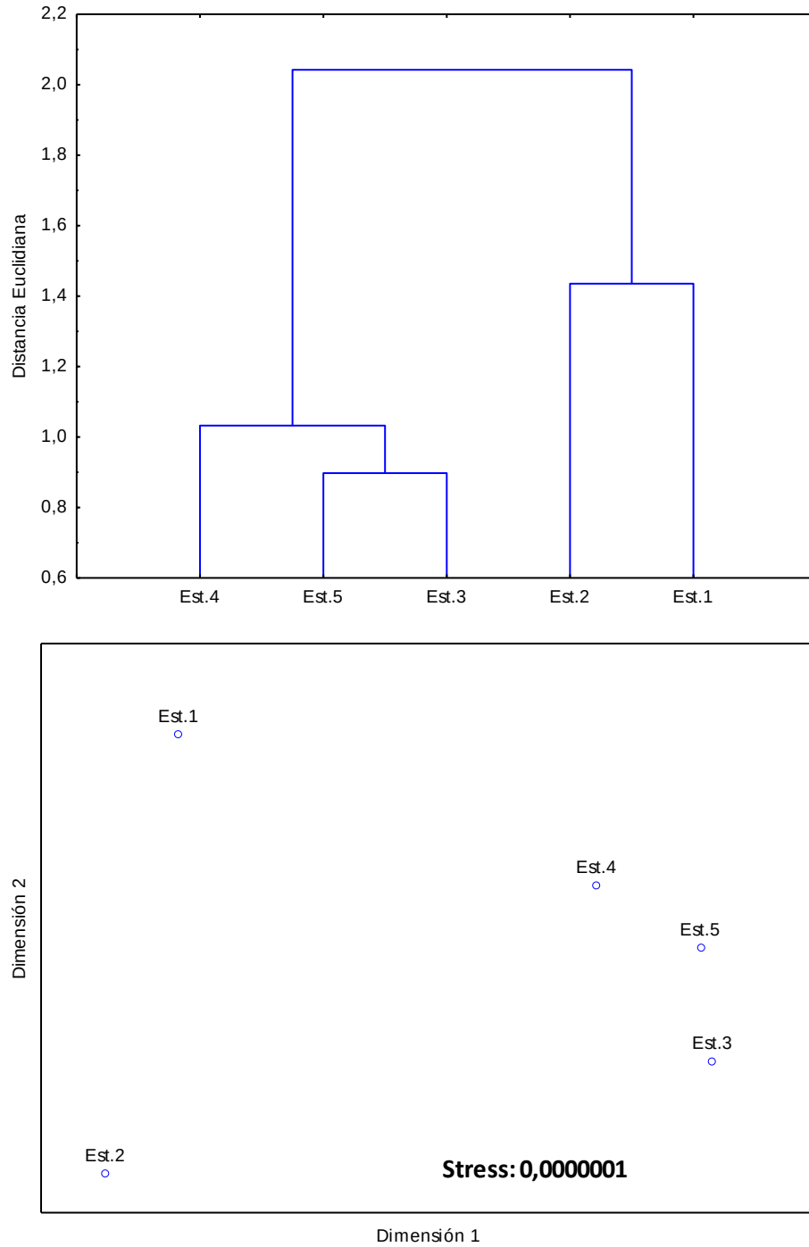
FIGURA 14. PUERTO MEJILLONES. Análisis multidimensional de las variables químicas en biota submareal (moluscos bivalvos) en las estaciones submareales de muestreo del PSM. MONITOREO MARZO 2014.
