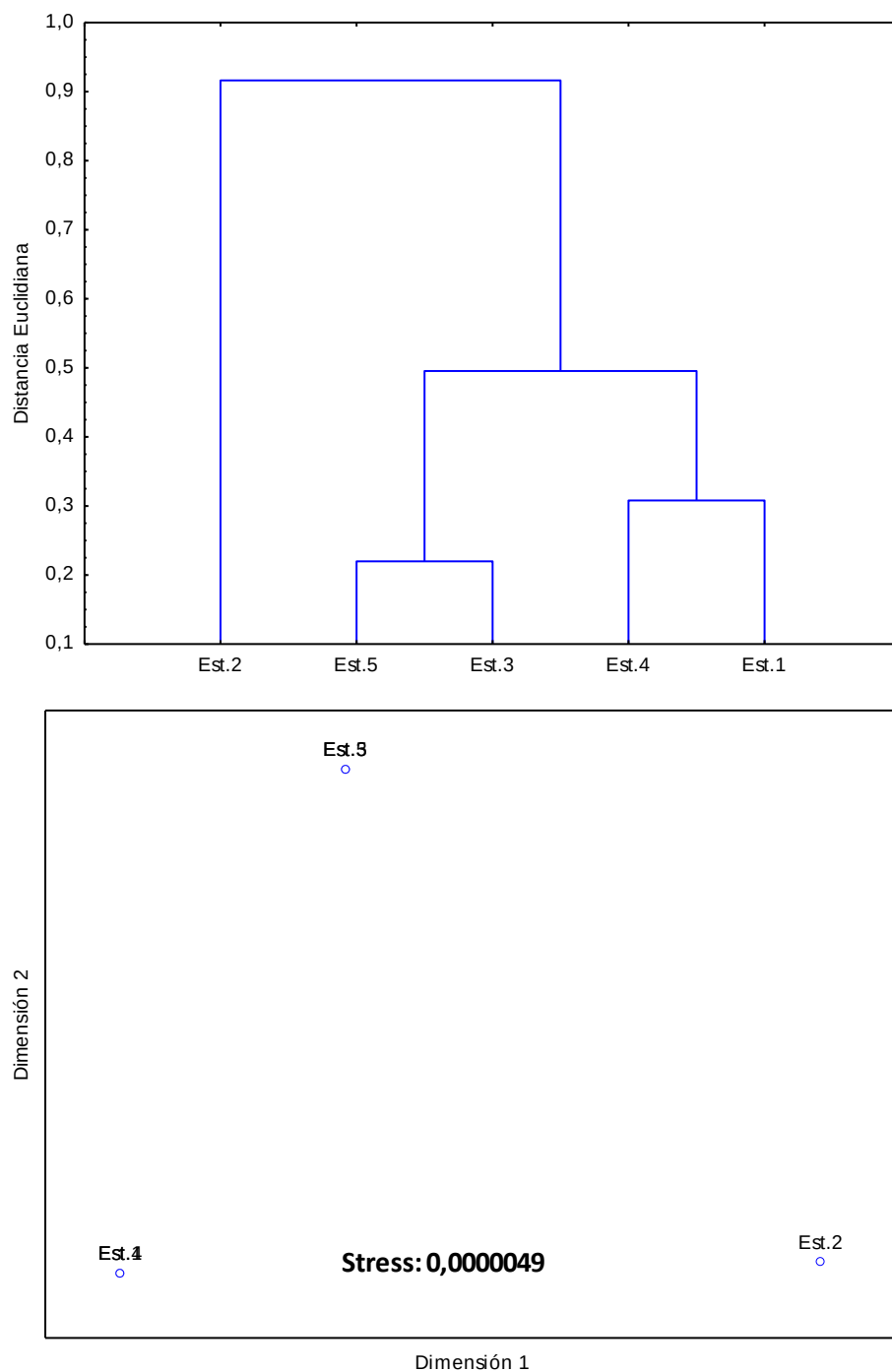
FIGURA 8. PUERTO MEJILLONES. Análisis multidimensional de las variables químicas en el estrato SUPERFICIAL de la columna de agua en las estaciones de muestreo del PSM. MONITOREO MARZO 2014.
