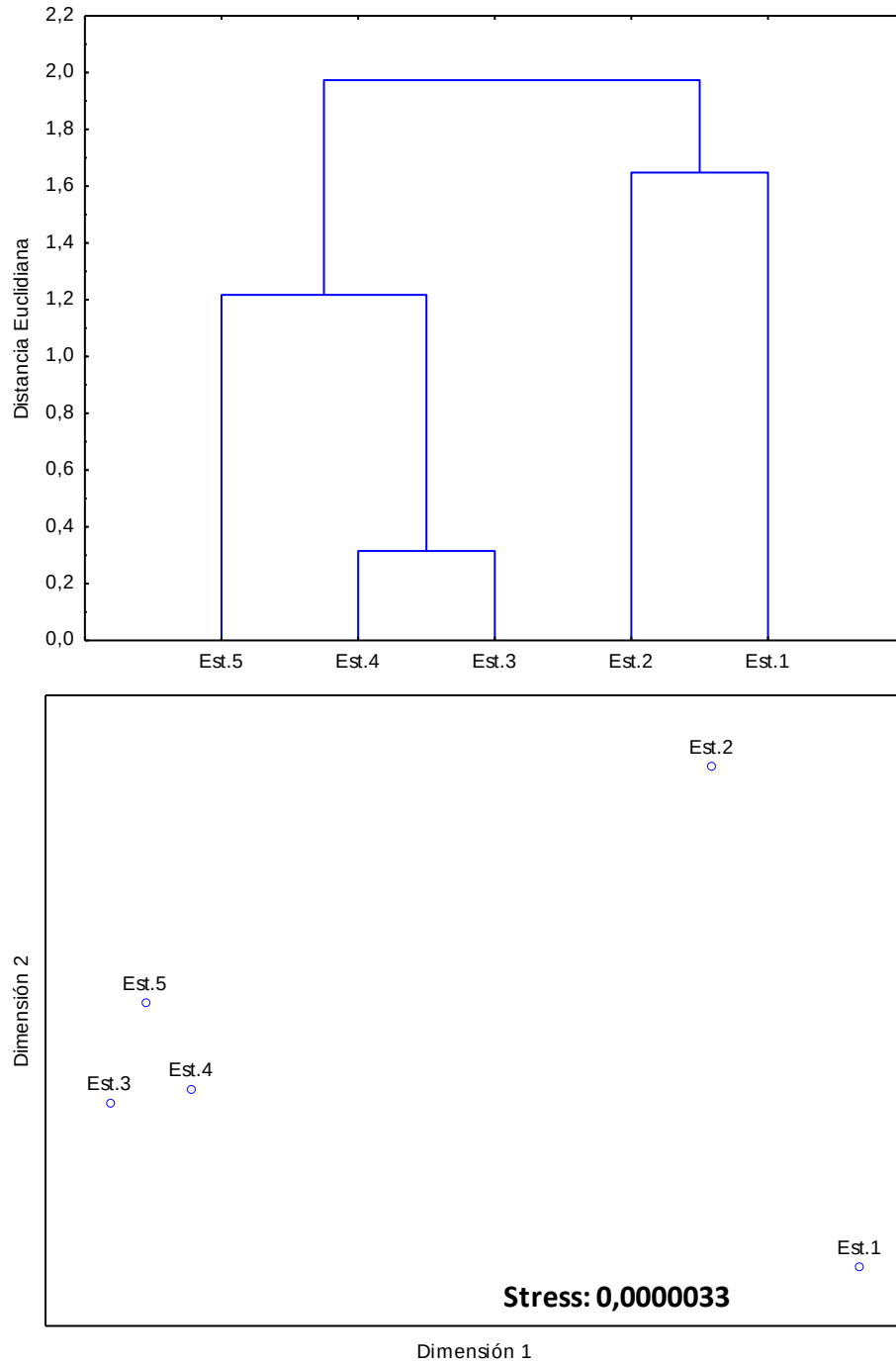
FIGURA 12. PUERTO MEJILLONES. Análisis multidimensional de las variables químicas en los sedimentos de las estaciones submareales en el muestreo del PSM. MONITOREO MARZO 2014.
