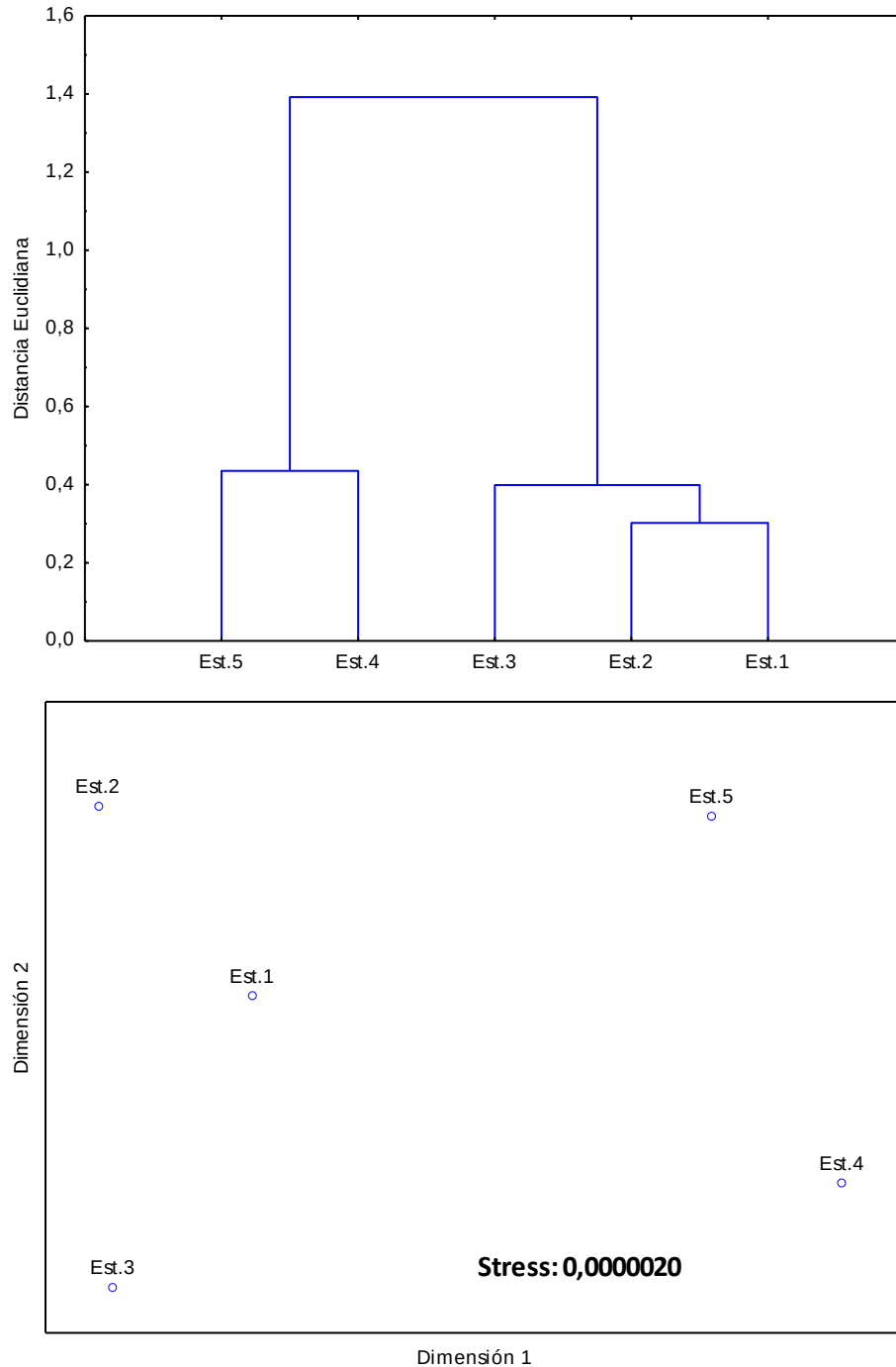
FIGURA 9. PUERTO MEJILLONES. Análisis multidimensional de las variables químicas del estrato PROFUNDO de la columna de agua en las estaciones de muestreo del PSM. MONITOREO MARZO 2014.
