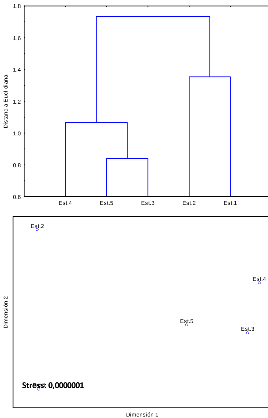
FIGURA 14. PUERTO MEJILLONES. Análisis multidimensional de las variables químicas en biota submareal (moluscos bivalvos) en las estaciones submareales de muestreo del PSM. MONITOREO AGOSTO 2015.
