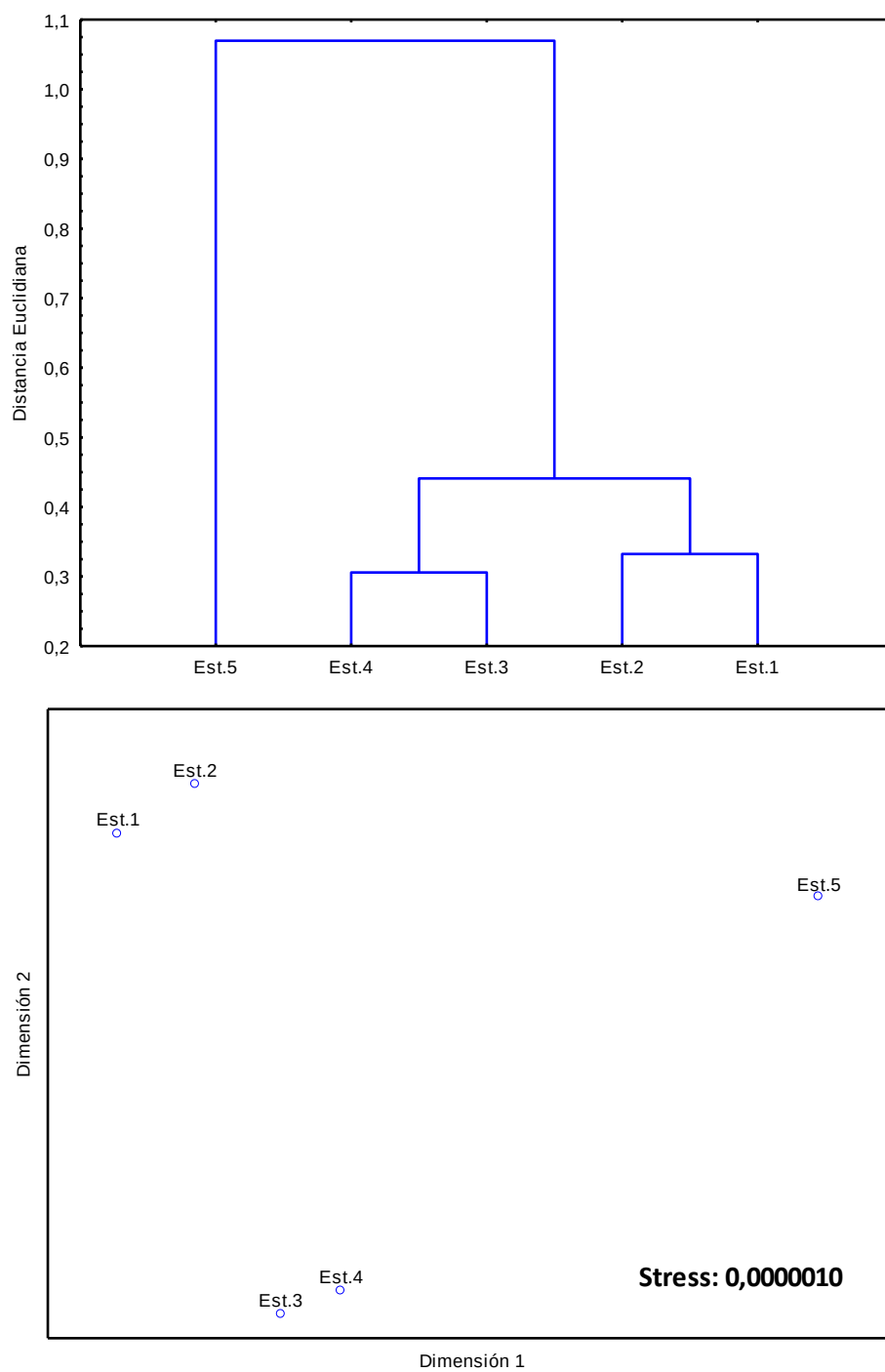
FIGURA 9. PUERTO MEJILLONES. Análisis multidimensional de las variables químicas del estrato PROFUNDO de la columna de agua en las estaciones de muestreo del PSM. MONITOREO AGOSTO 2015.
