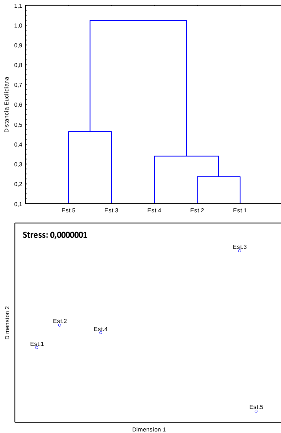
FIGURA 8. PUERTO MEJILLONES. Análisis multidimensional de las variables químicas en el estrato SUPERFICIAL de la columna de agua en las estaciones de muestreo del PSM. MONITOREO AGOSTO 2015.
