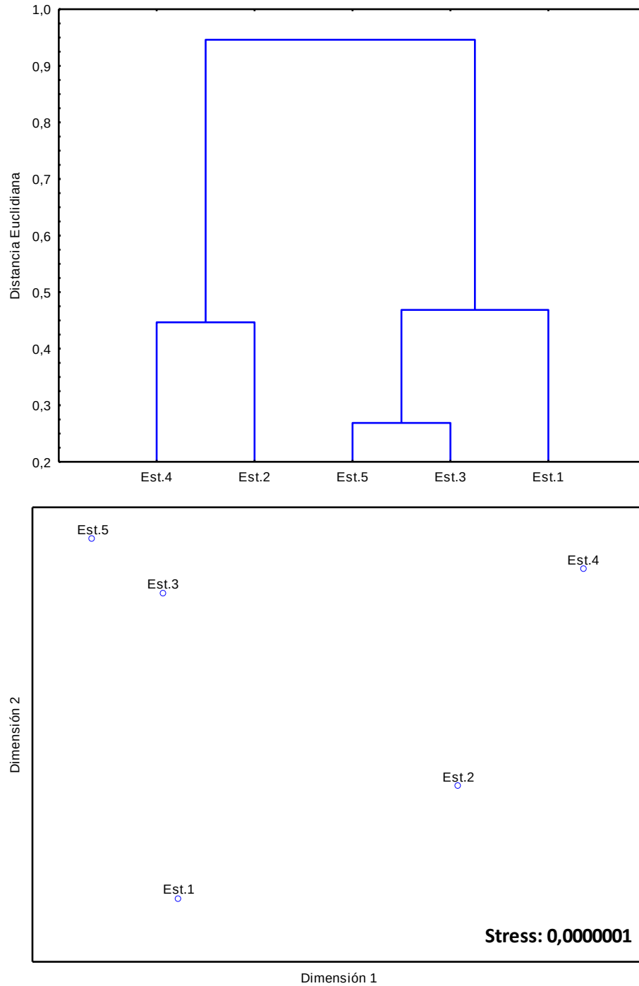
FIGURA 13. PUERTO MEJILLONES. Análisis multidimensional de las variables químicas en biota intermareal ( Emerita analoga ) en las transectas intermareales de muestreo del PSM. MONITOREO AGOSTO 2015.
