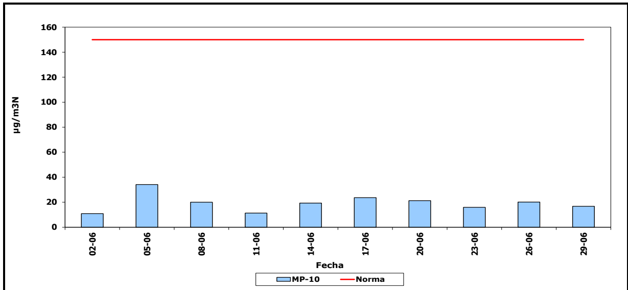
Gráfico N° 1 Concentración de Material Particulado Respirable MP-10 Estación Puerto Mejillones, Junio 2020
